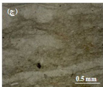
شکل ۷. الف: مادستون با فابریک چشم پرنده‌ای، ب: مادستون با قالب بلورهای تبخیری - پهنه جزر و مدی (T 1 ) ج: باندستون استروماتولیتی - پهنه جزر و مدی (T 2 ) (نورپلاریزه)
