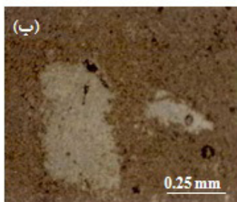
شکل ۷. الف: مادستون با فابریک چشم پرنده‌ای، ب: مادستون با قالب بلورهای تبخیری - پهنه جزر و مدی (T 1 ) ج: باندستون استروماتولیتی - پهنه جزر و مدی (T 2 ) (نورپلاریزه)
