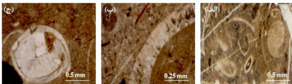
شکل ۵. الف: بایوکلاستیک وکستون - پکستون - لاگون (L 1 ) ب: بایوکلاستیک وکستون با فسیل شکم‌پایان - لاگون (L 2 ) ج: بایوکلاستیک وکستون - لاگون (L 3 ) (نورپلاریزه)
