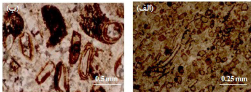
شکل ۴. الف: بایوکلاستیک گریستون - سد (S 1 ) (نورپلاریزه) ب: ائیدگریستون - سد (S 2 ) (نور طبیعی)
