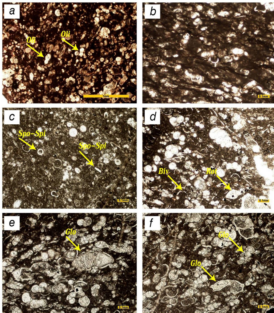
شکل ۴. تصاویر میکروسکوپی رخشاره‌های رسوبی زیرمحیط دریای باز سازند ایلام: (a,b,c) ریزرخساره وکستون-پکستون اُلیگوستژینا اسپیکول اسفنج‌دار، (PPL) در ژرفای ۴۳۰۵ متری از چاه شماره ۲ میدان قلعه نار. (d,e,f) ریزرخساره وکستون-پکستون بایوکلاست‌دار، (PPL) ژرفای ۴۲۸۵ متری از چاه شماره ۳ میدان قلعه نار
