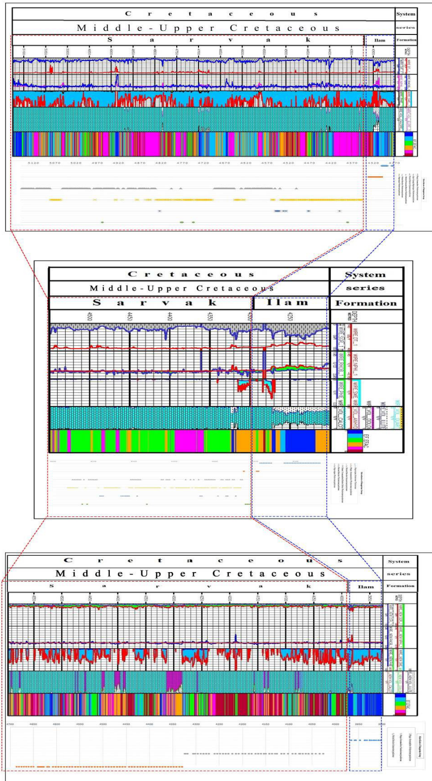
شکل ۹. مقایسه رخساره‌های الکتریکی و ریزرخساره‌های رسوبی در سه چاه مورد بررسی از میدان نفتی قلعه نار
