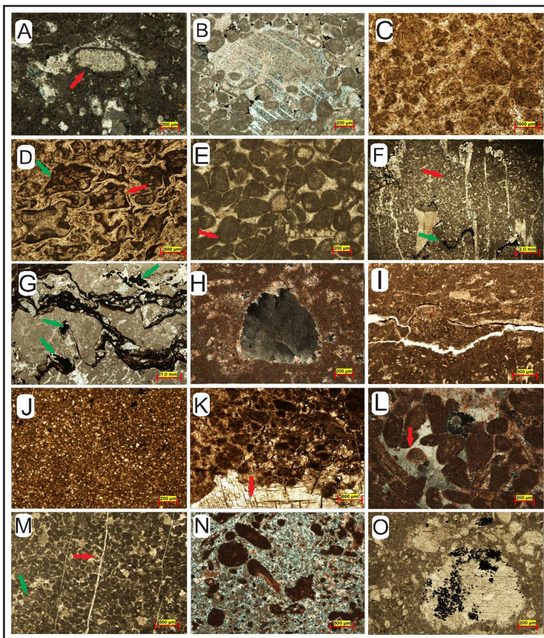
شکل ۷. A) میکربیتی‌شدن؛ B) سیمانی‌شدن هم‌محور و فراگیر؛ C) نوریختی افزایشی در آئیدها و خمیره؛ D) تغییر شکل بیوکلاست‌ها (پیکان سرخ) و شکستگی سیمان هم‌ستبراً پیرامون دانه‌ها (پیکان سبز)؛ E) انواع همبری‌های کاو-کوژ و مضرس؛ F) استیلولیتی‌شدن و دولومیتی‌شدن همراه آن؛ G) استیلولیتی‌شدن و پیریت (پیکان سبز) و آغستگی‌های هیدروکربنی در سطوح آن؛ H) دولومیت زین‌اسبی به‌صورت پرکننده حفره (رنگ‌آمیزی با آلزارین سرخ)؛ I) تخلخل در راستای استیلولیت؛ J) دولومادستون؛ K) دولومیت درشت‌بلور زین‌اسبی (در واکنش با آلزارین سرخ، رنگ نگرفته است)؛ L) دولومیت زین‌اسبی به‌صورت پرکننده تخلخل‌های میان‌دانه‌ای (رنگ‌آمیزی با آلزارین سرخ)؛ M) شکستگی‌های (پیکان سرخ) قطع‌کننده سطح استیلولیت (پیکان سبز)؛ N) سیلیسی‌شدن؛ O) پیریتی‌شدن به‌صورت جانشینی اسکلت اکینودرم
