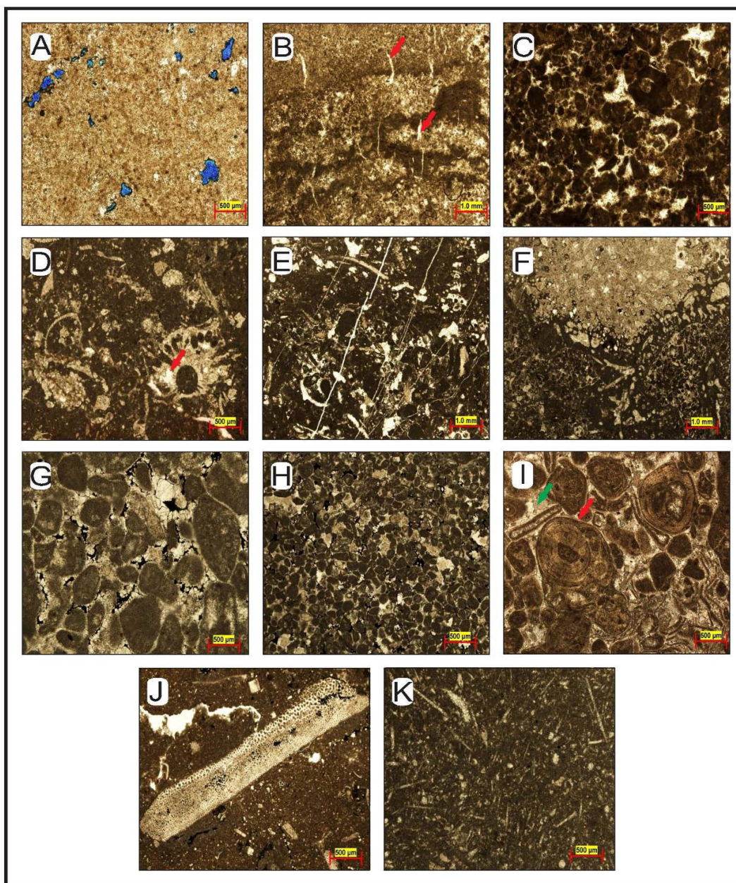
شکل ۳. A) ریزرخساره گل‌سنگ آهکی/دولومیتی؛ B) ریزرخساره باندستون استرماتولیتی دارای ترک گلی پر شده با کلسیت اسپاری؛ C) ریزرخساره پکستون-گرینستون پلوییدی؛ D) ریزرخساره مادستون/وکستون بیوکلاستی؛ انحلال و تخلخل قالبی ایجاد شده عمدتاً با سیمان پر شده؛ E) ریزرخساره پکستون پلوییدی بیوکلاستی؛ F) ریزرخساره فلوتستون استرماتوپلوییدی پلوییدی؛ G) ریزرخساره گرینستون پلوییدی اینتراکلاستدار؛ H) ریزرخساره گرینستون پلوییدی بیوکلاستی؛ I) ریزرخساره گرینستون آبییدی پلوییدی؛ سیمان هم‌سترا (پیکان سرخ) و هم‌بعد میان‌دانه‌ای (پیکان سبز)؛ J) ریزرخساره وکستون بیوکلاستی؛ K) وکستون بیوکلاستی
