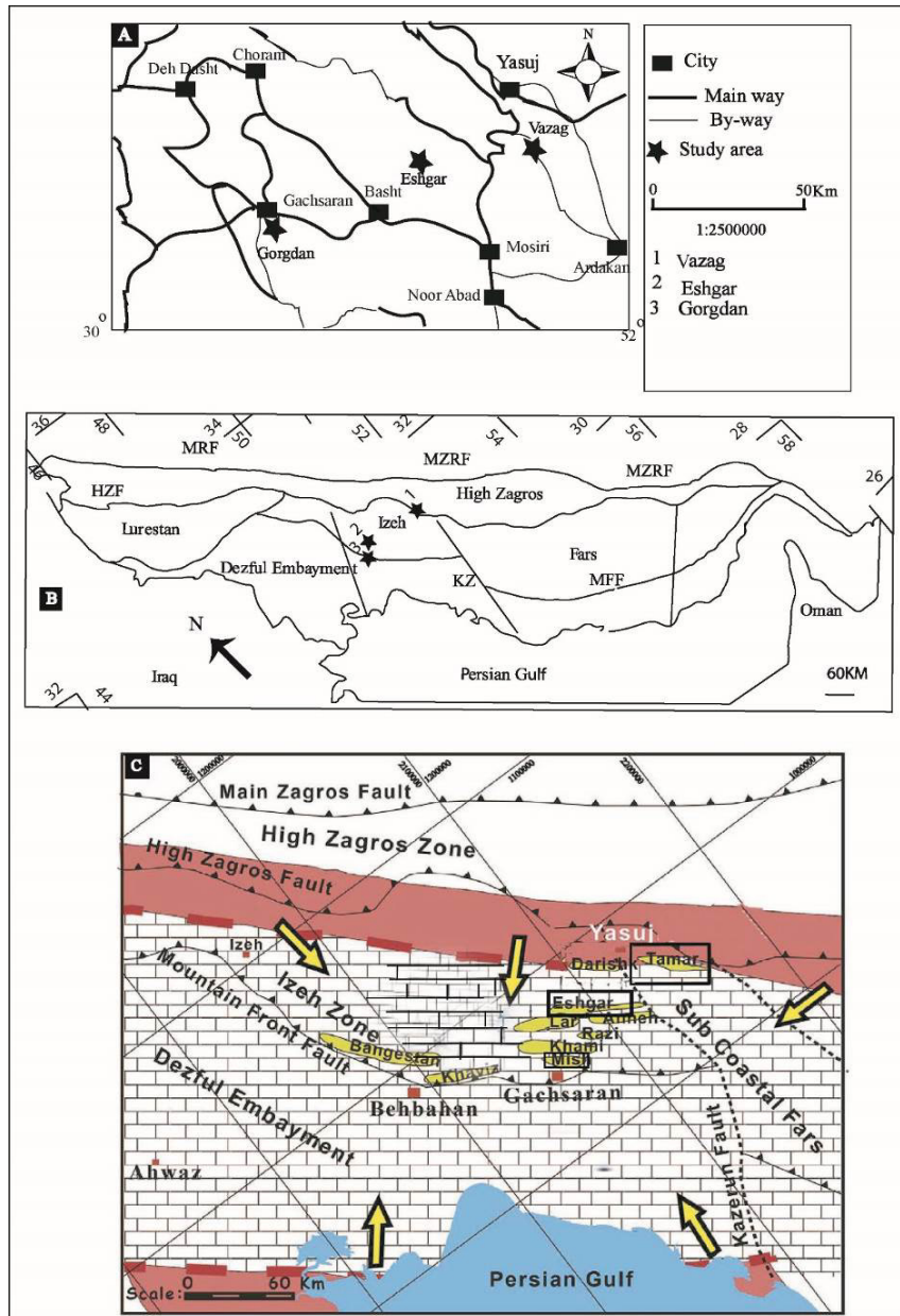
شکل ۲. نقشه راه‌ها و زمین‌شناسی منطقه مورد پژوهش. A: راه‌های دسترسی به رخنمون‌های مورد پژوهش (برگرفته از نقشه راه‌های ایران ۱۳۸۴). B: جایگاه زمین‌شناسی ساختاری حوضه زاگرس C: حوضه اینتراشلف آسماری. پیکان‌های زرد مشخص‌کننده پیشروی رسوبات الیگو- میوسن به سمت بخش‌های ژرف حوضه است. مستطیل سیاه جایگاه رخنمون‌های مورد پژوهش. نواحی زرد رنگ تاقدیس‌های منطقه (الله کرم پوردیل ۲۰۱۸).
