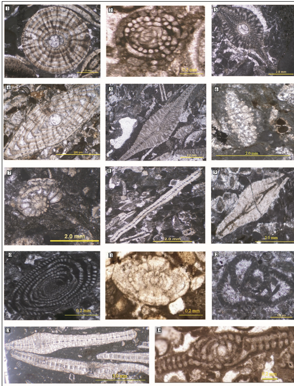
شکل ۱۳. تصویرهایی از فسیل‌های شناسایی شده در رخنمون‌های وزگ، اشگر و گرگان.
