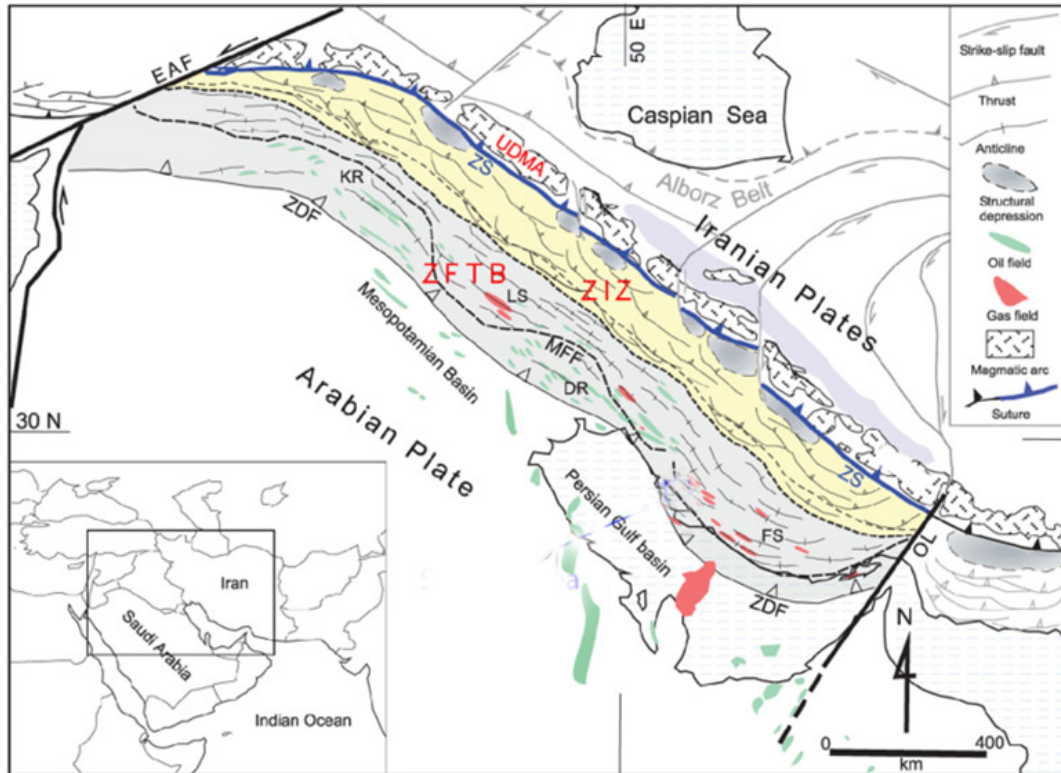
شکل ۱. گسترش کمر بند زاگرس، تقسیمات و مرزهای محدود کننده آن UDMA: مجموعه ماگمایی ارومیه- دختر، EAF: گسل خاوری آناتولی، ZDF: جبهه تغییر شکل زاگرس، ZS: خط درز زاگرس، ZTZ: زون راندگی زاگرس، ZIZ: زون روی هم چین خورده، ZFTB: زون رورانده- چین خورده زاگرس، OL: خط عمان (علوی، ۲۰۰۷).
