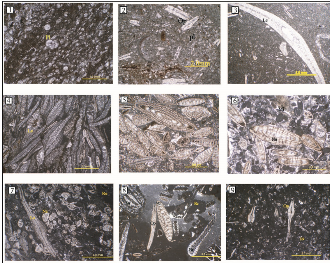
شکل ۱۴. پلانکتونیک فرامینیفرای وکستون/پکستون. نمونه ۲ رخنمون گرگدان. ۲- بایوکلاستیک پلانکتونیک فرامینیفرای وکستون/پکستون. نمونه ۱۹ رخنمون اشگر. ۳- بایوکلاستیک لپیدوسیکیلینا وکستون/فلوتستون. نمونه ۲۳ رخنمون اشگر. ۴- بایوکلاستیک لپیدوسیکیلینا/نومولیتیده پکستون/رودستون. نمونه ۱۰ رخنمون گرگدان. ۵- بایوکلاستیک لپیدوسیکیلینا/نومولیتیده پکستون/رودستون. نمونه ۴۹ رخنمون وزگ. ۶- بایوکلاستیک میلیولید نومولیتیده پکستون/گرینستون. نمونه ۳۱ رخنمون وزگ. ۷- بایوکلاستیک فرامینیفرای منفذدار کورالیناسه‌آ نئوروتالیا پکستون/رودستون. نمونه ۲۶ رخنمون گرگدان. ۸- بایوکلاستیک فرامینیفرای منفذدار کورالیناسه‌آ بریوزوئر پکستون/فلوتستون. نمونه ۴ رخنمون وزگ. ۹- بایوکلاستیک فرامینیفرای منفذدار کورالیناسه‌آ پکستون/رودستون. نمونه ۹ رخنمون گرگدان.
