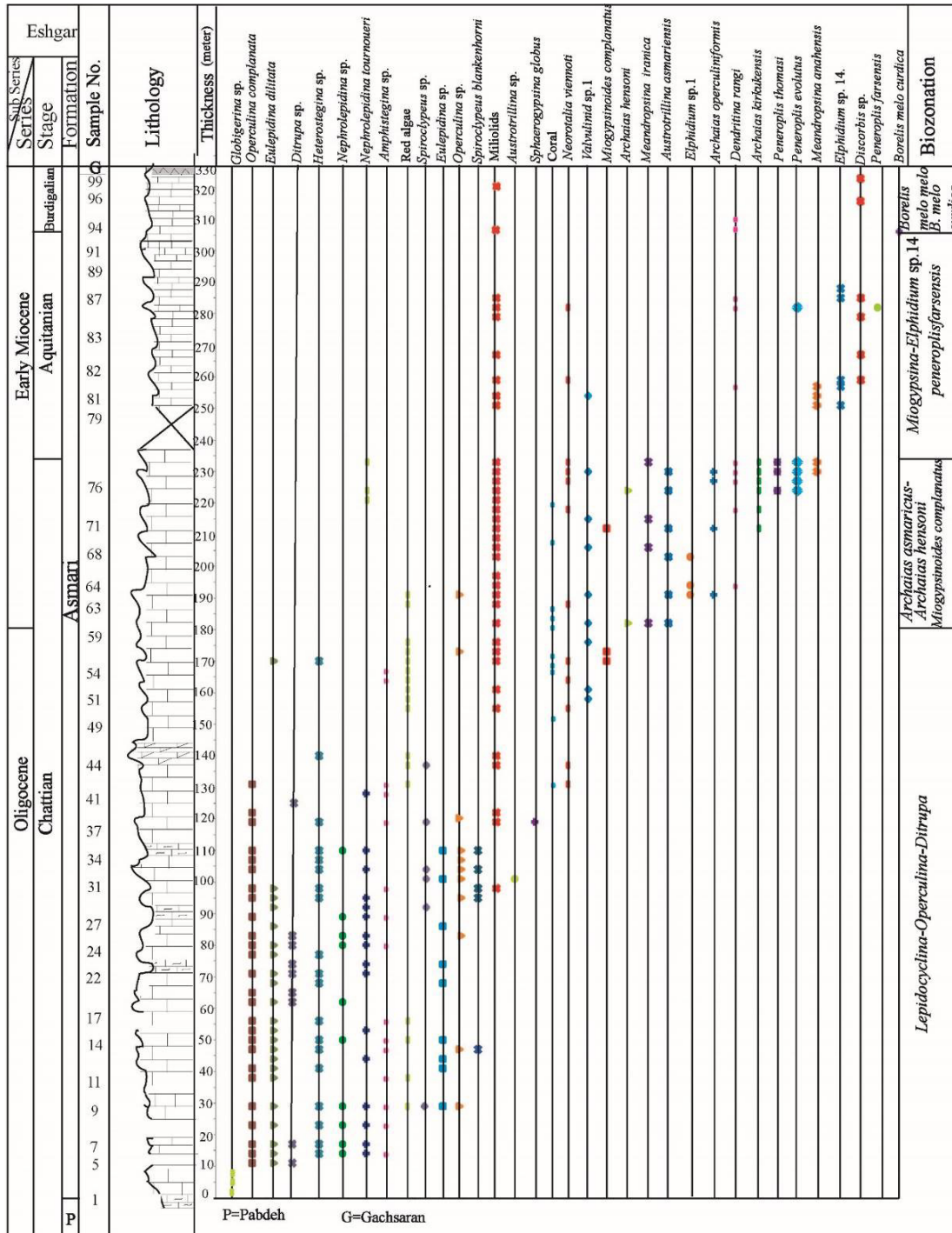
شکل ۴. ستون گسترش چینهننگاری زیستی سازند آسماری در رخنمون اشگر بر مبنای چینهننگاری زیستی لارسن و همکاران (۲۰۰۹)
