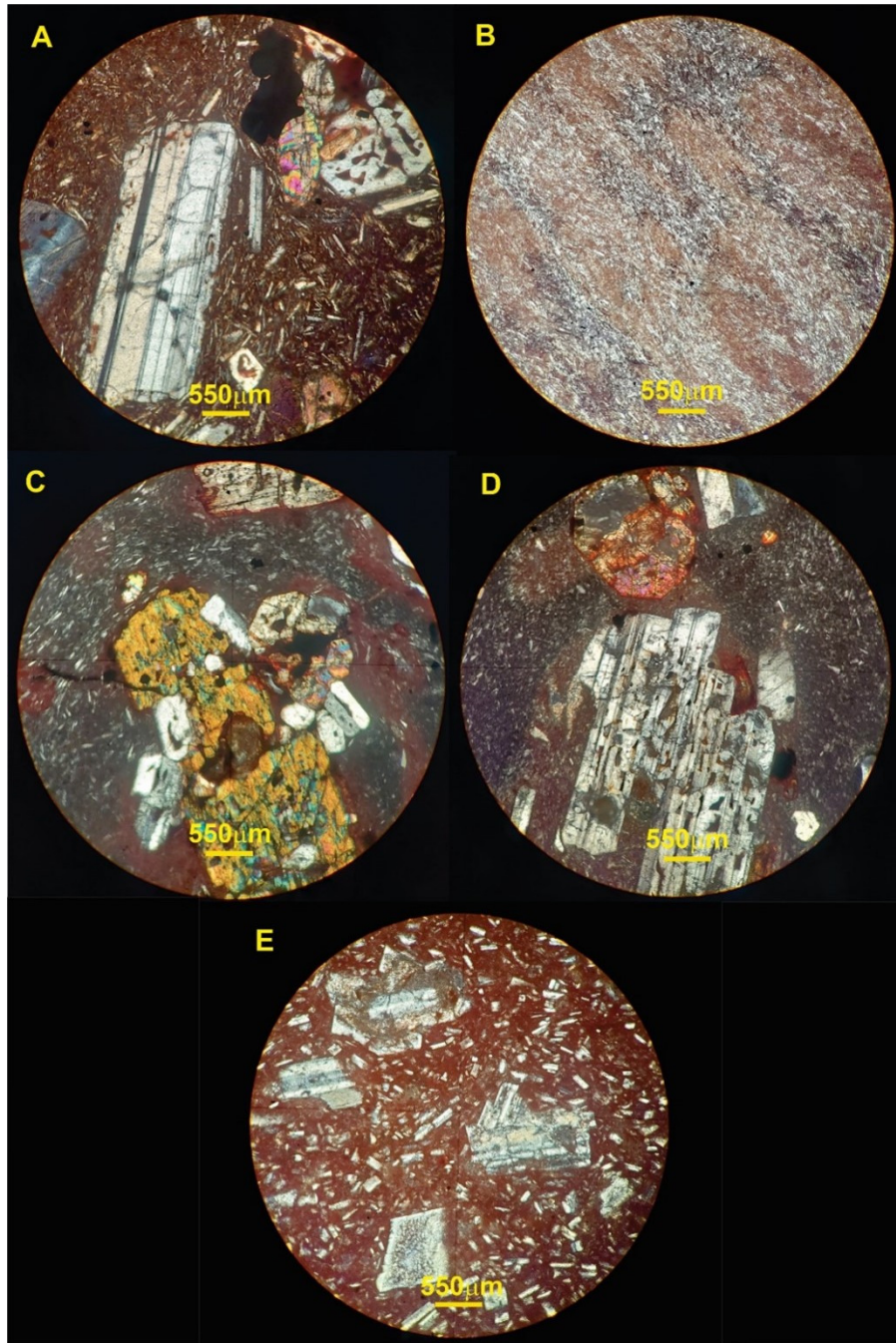
شکل ۱۲. تصاویر میکروسکوپی (XPL) قطعات گراولی پراکنده در اطراف محوطه و دیواره کانال رودخانه مجاور محوطه. (A) آندزیت بازالتی، (B) بازالت، (C) پیروکسن آندزیت با بافت گلومروپورفیری همراه با پلاژیوکلازهای با بافت غربالی، (D) آندزیت با پلاژیوکلازهای با بافت غربالی، (E) آندزیت.
