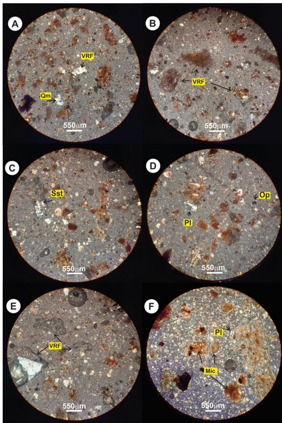
شکل ۱۰. تصاویر میکروسکوپی (نور XPL) از اجزاء تشکیل دهنده نمونه‌های خاک سطحی محوطه کهنک. کوارتز تک‌بلور (Qm)، کوارتز چند-بلور (Qp)، پلاژیوکلاز (Pl)، خرده‌سنگ‌های ولکانیکی حدواسط و مافیک (VRF)، خرده‌سنگ رسوبی ماسه‌سنگی (Sst) و قطعات میکریتی کربناته (Mic) در تصاویر مشخص شده است.
