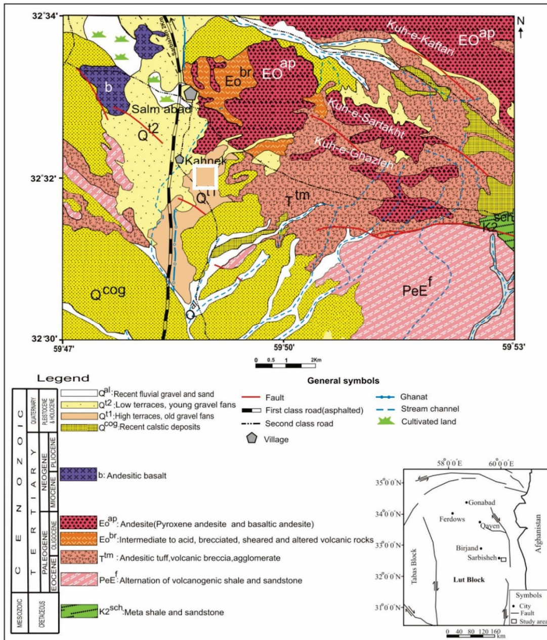
شکل ۱۴. نقشه زمین‌شناسی محدوده مورد مطالعه در جنوب سریش (برگرفته از گودرزی و همکاران، ۱۳۹۳). موقعیت محدوده مورد مطالعه در نقشه ساده بلوک لوت (کریم‌پور و همکاران، ۲۰۱۱) با علامت مستطیل نشان داده شده است. موقعیت محوطه باستانی کهنک نیز با مربع سفیدرنگ مشخص شده است.
