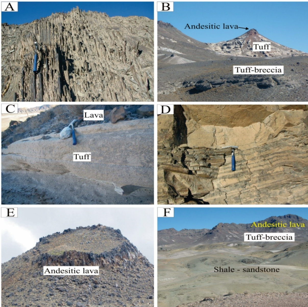
شکل ۱۵. A) نمای از شیل و ماسه‌سنگ‌های دگرگون‌شده در جنوب شرق سریشه، دید به سوی شمال غرب، B و C) حضور گدازه‌های آندزیتی بر روی توف‌ها در جنوب شرق سریشه، دید به سوی شمال شرق، D) لیتیک توف دربرگیرنده شیشه آتشفشانی و دارای حالت نواری در جنوب شرق سریشه، E) رخنمون واحدهای گدازه‌های آندزیتی در بخش‌های مرکزی و شمال شرق سلم‌آباد به صورت گنبدهایی با ساخت توده‌ای و گاهی ستونی، دید به سوی شمال شرق، F) نمایی از قرارگیری گدازه و آذرآوری‌ها بر روی شیل و ماسه‌سنگ در شرق روستای کهنک، دید به سوی شمال شرق (گودرزی و همکاران، ۱۳۹۳).
