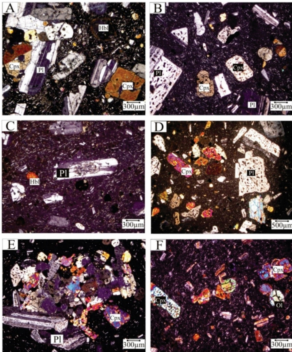
شکل ۱۶. تصاویر میکروسکوپی از آندزیت‌های منطقه مورد مطالعه (نور XPL). A) بافت پورفیری با زمینه میکرولیتی، B) بافت‌های غیرتعادلی نظیر بافت غربالی در پلاژیوکلازها و حضور کلینوپیروکسن‌های شکل‌دار تا نیمه‌شکل‌دار، C) بافت پورفیری با زمینه میکرولیتی شیشه‌ای، هورنبلندهای نیمه‌شکل‌دار و دگرسانی بخش مرکزی پلاژیوکلاز به کربنات، D) بافت غربالی در پلاژیوکلاز و فراوانی پیروکسن در پیروکسن آندزیت‌ها، E) تجمعات پلاژیوکلاز و پیروکسن و تشکیل بافت گلومروپورفیری در پیروکسن آندزیت‌ها، F) الیوین ریزبلور به همراه کلینوپیروکسن در آندزیت‌های بازالتی (گودرزی و همکاران، ۱۳۹۳).
