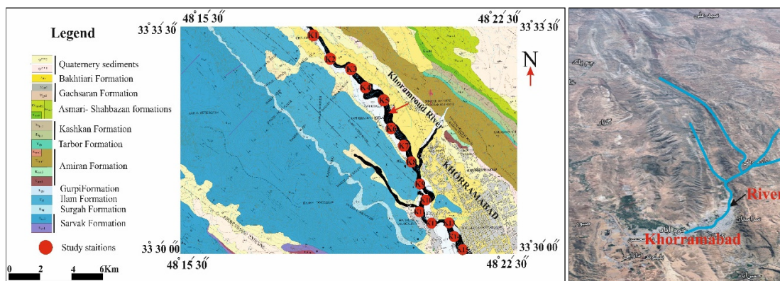
شکل ۲. نقشه زمین‌شناسی منطقه مورد مطالعه (سازمان زمین‌شناسی کشور، ۲۰۱۱) به همراه تصویر ماهواره‌ای گسترش حوزه آبریز رودخانه خرم‌رود. مکان‌های نمونه‌برداری روی شکل با دایره قرمز رنگ و با کدهای K1 تا K15 نشان داده شده‌اند.
